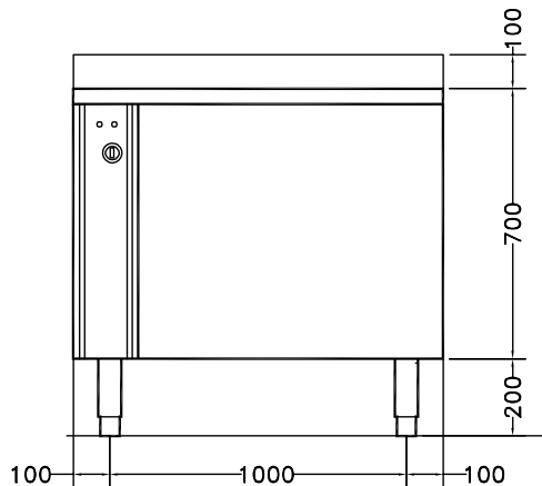
Zij aanzicht
